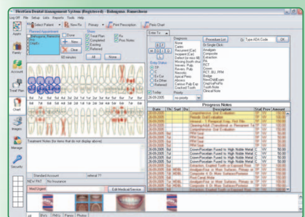
Chart Module
