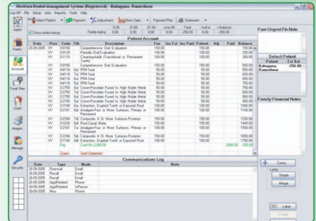
Accounts Module
